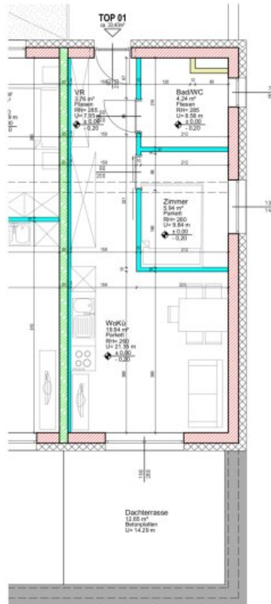
Planausschnitt 1.OBERGESCHOSS - Wohnung Planstand = Ausführungsplan M: 1:100
