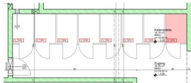
Planausschnitt KELLERGESCHOSS - Abteil TOP 01 - WEST Planstand = Ausführungsplan M: 1:100
