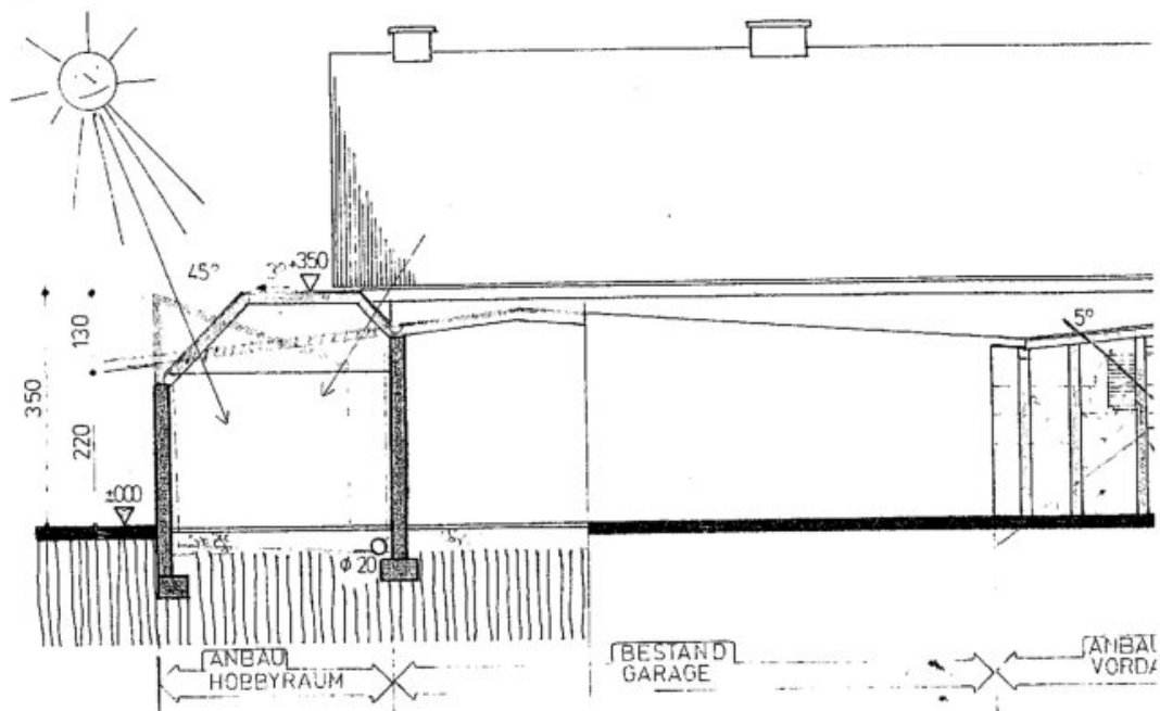
SNITT UND ANSICHT VON WESTEN
