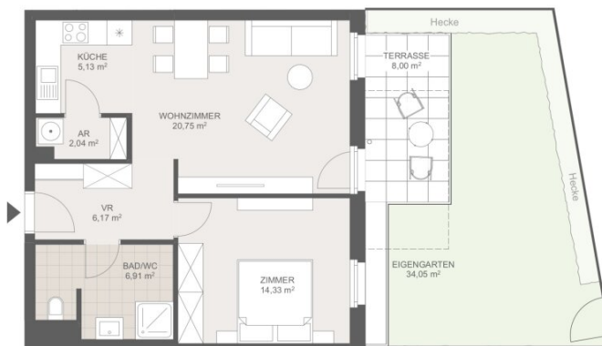
Grundriss 1:100
