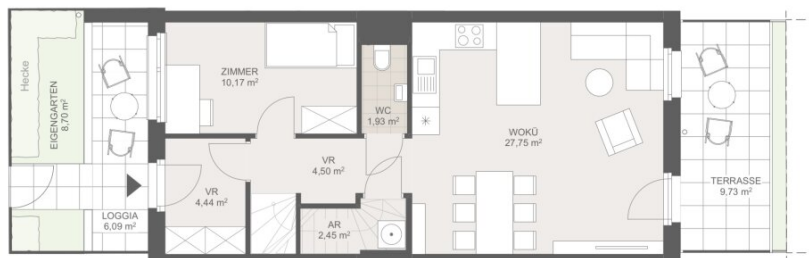
Grundriss 1:100
