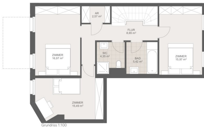
Grundriss 1:100
