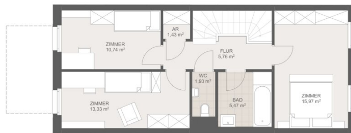
Grundriss 1:100
