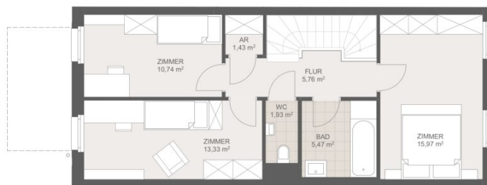
Grundriss 1:100
