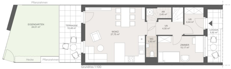
Grundriss 1:100
