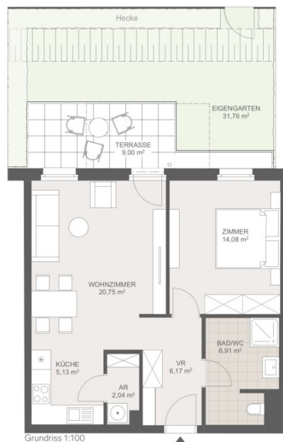
Grundriss 1:100
