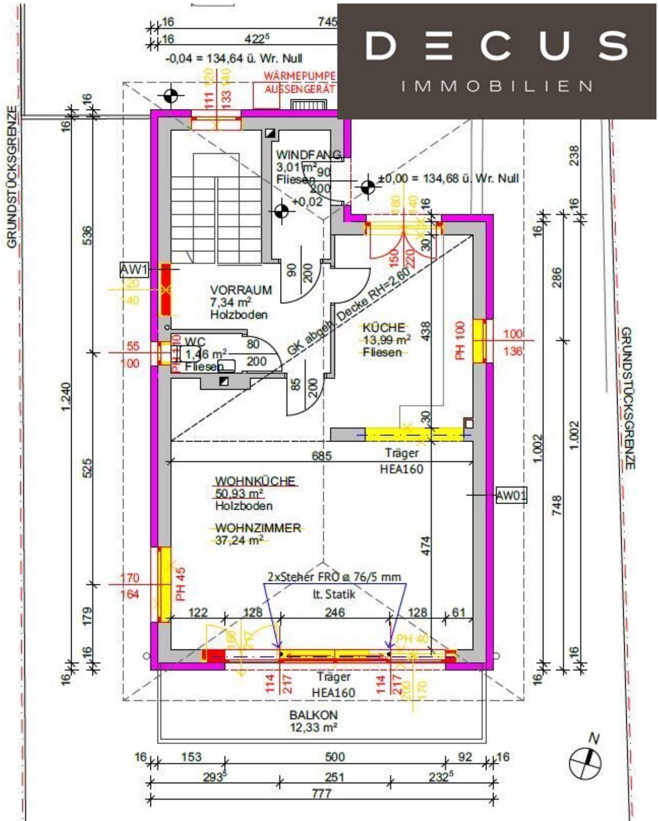
ERDGESCHOSS
