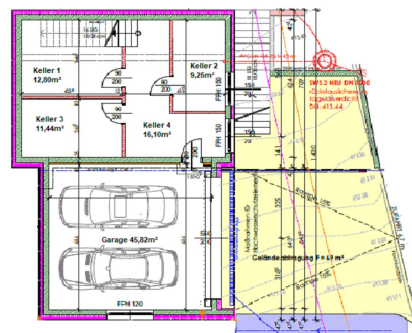
Grundriss Kellergeschoss
