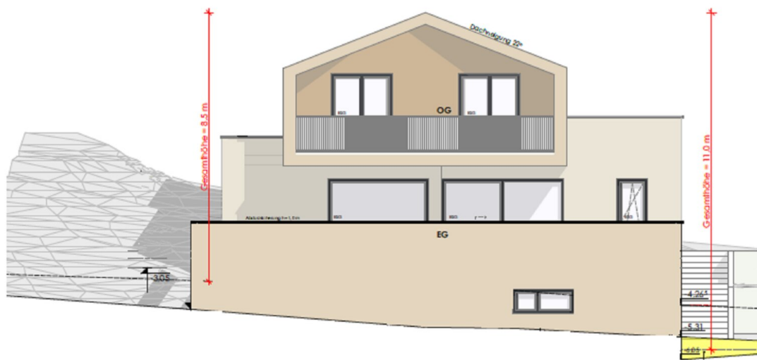
ANSICHT SÜDEN Haus A
