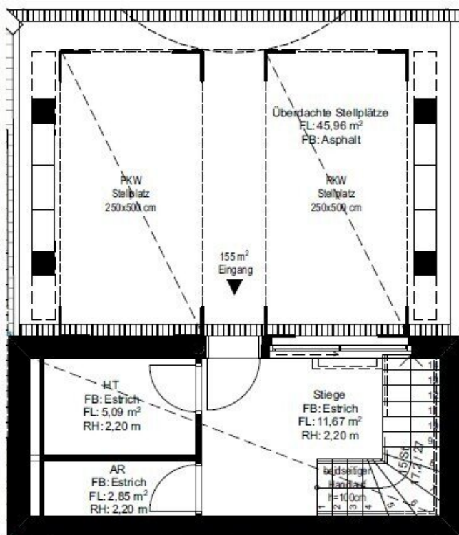
Kellergeschoss 1:100
