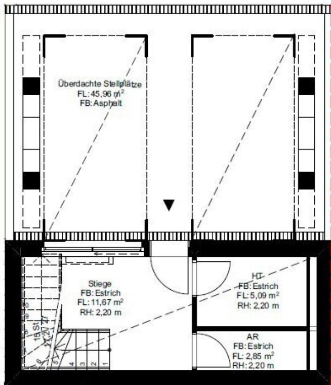
Kellergeschoss 1:100
