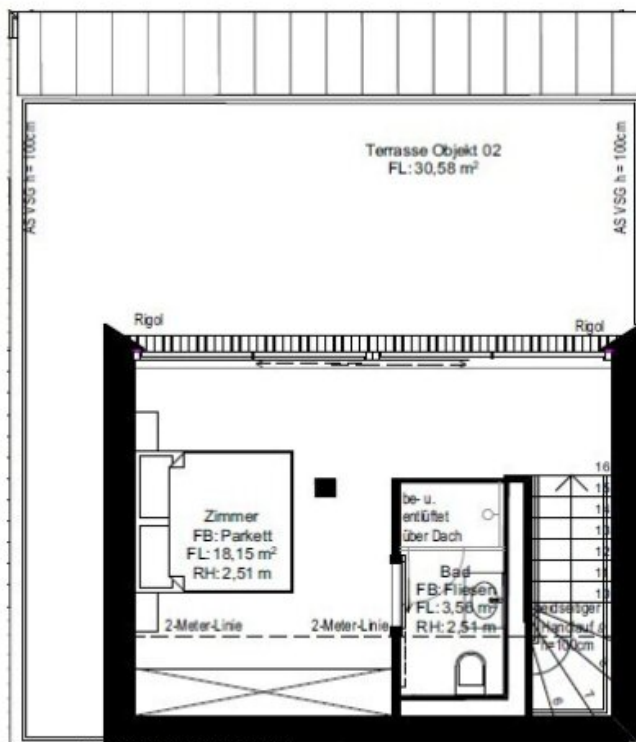
Dachgeschoss 1:100
