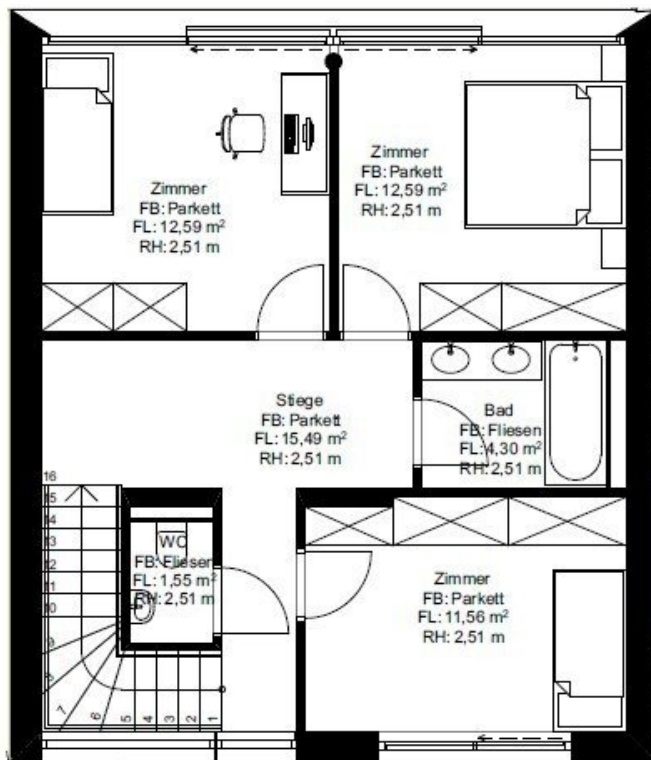
Obergeschoss 1:100
