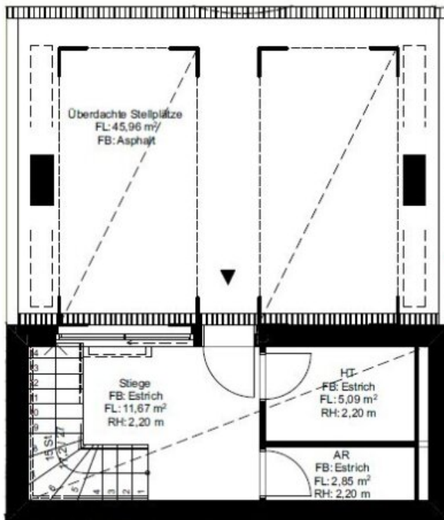
Kellergeschoss 1:100
