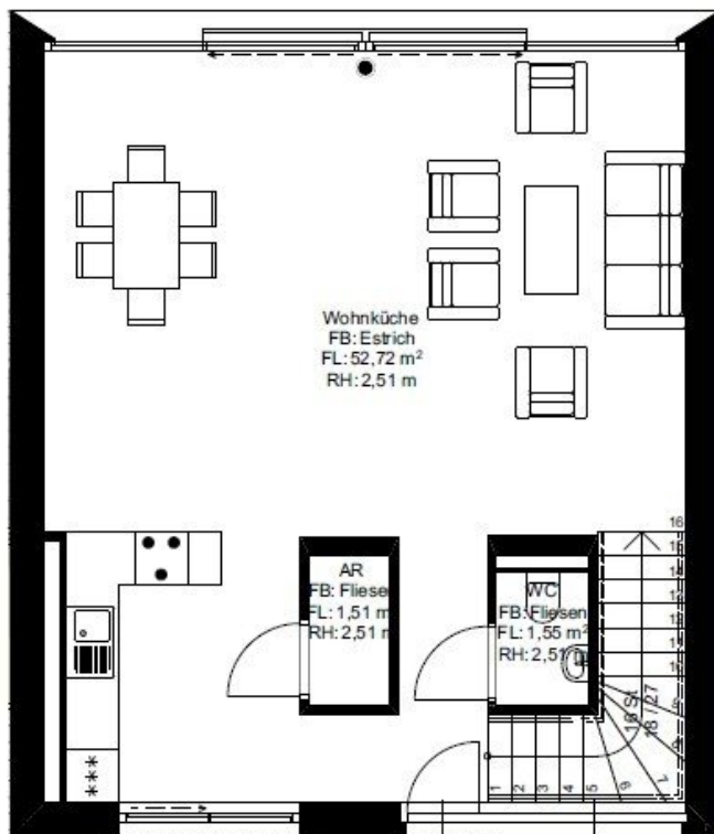
Erdgeschoss 1:100
