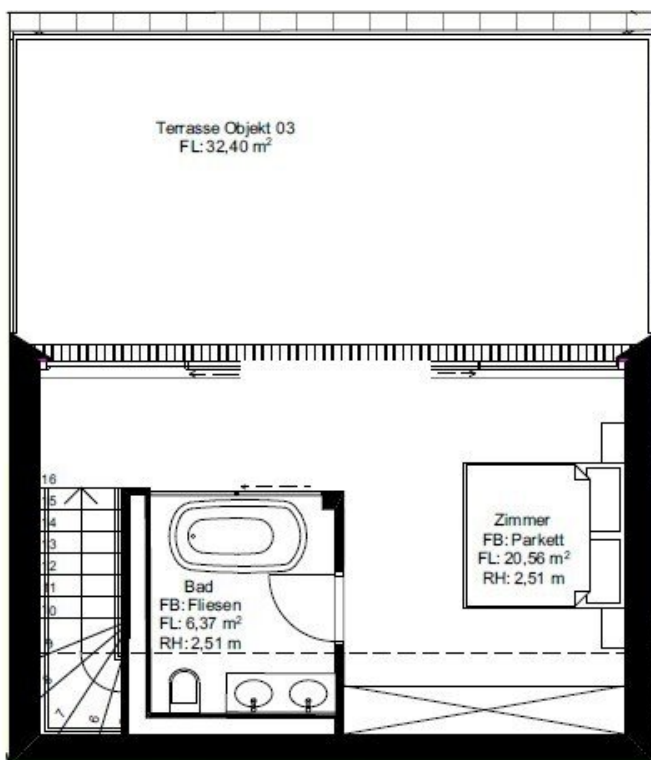
Dachgeschoss 1:100
