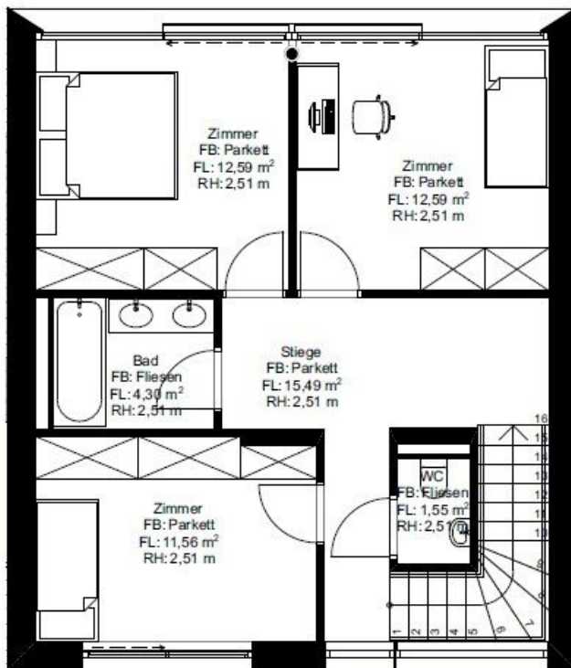
Obergeschoss 1:100
