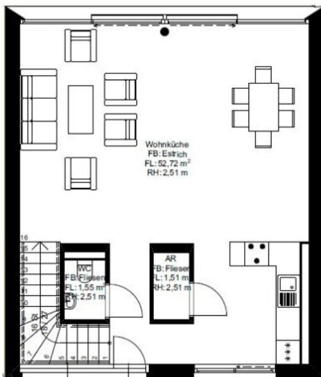
Erdgeschoss 1:100
