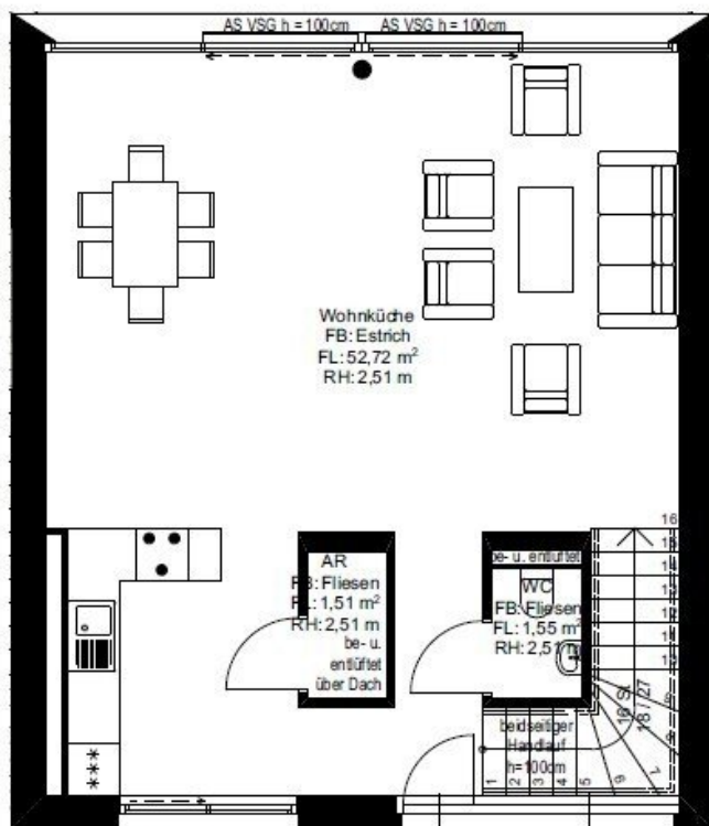
Erdgeschoss 1:100
