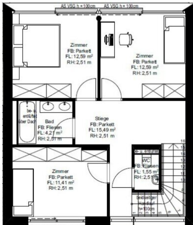
Obergeschoss 1:100
