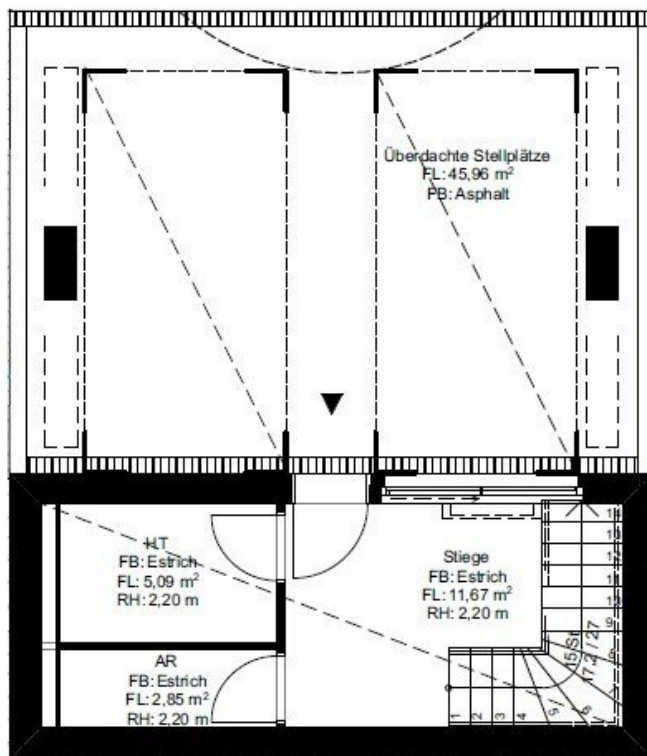
Kellergeschoss 1:100
