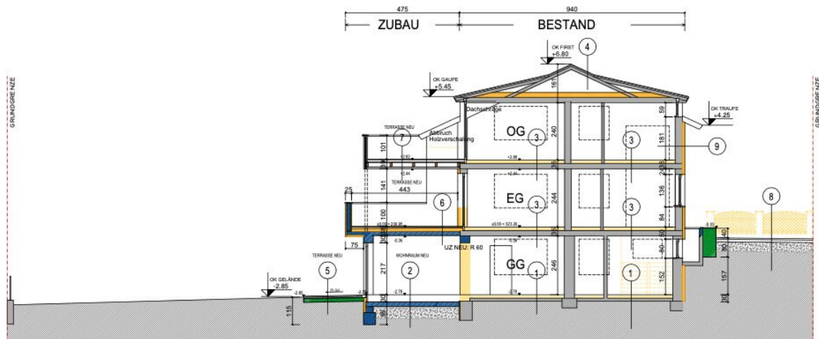
SCHNITT A-A
