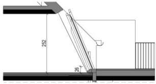
Schnitt 46 A
