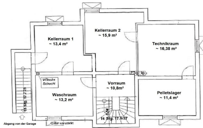
Kellergeschoss Skizze
