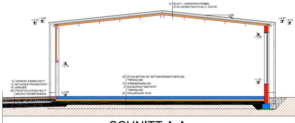
SCHNITT A-A
