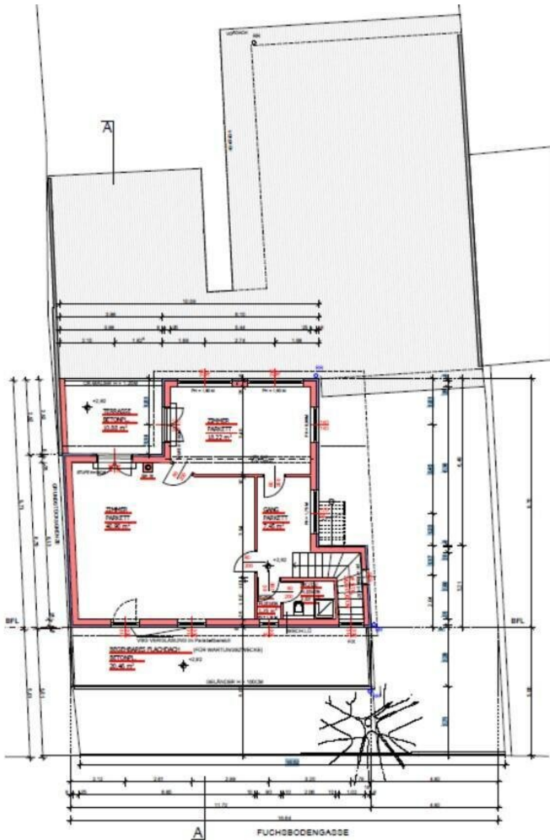
GRUNDRISS OBERGESCHOSS
