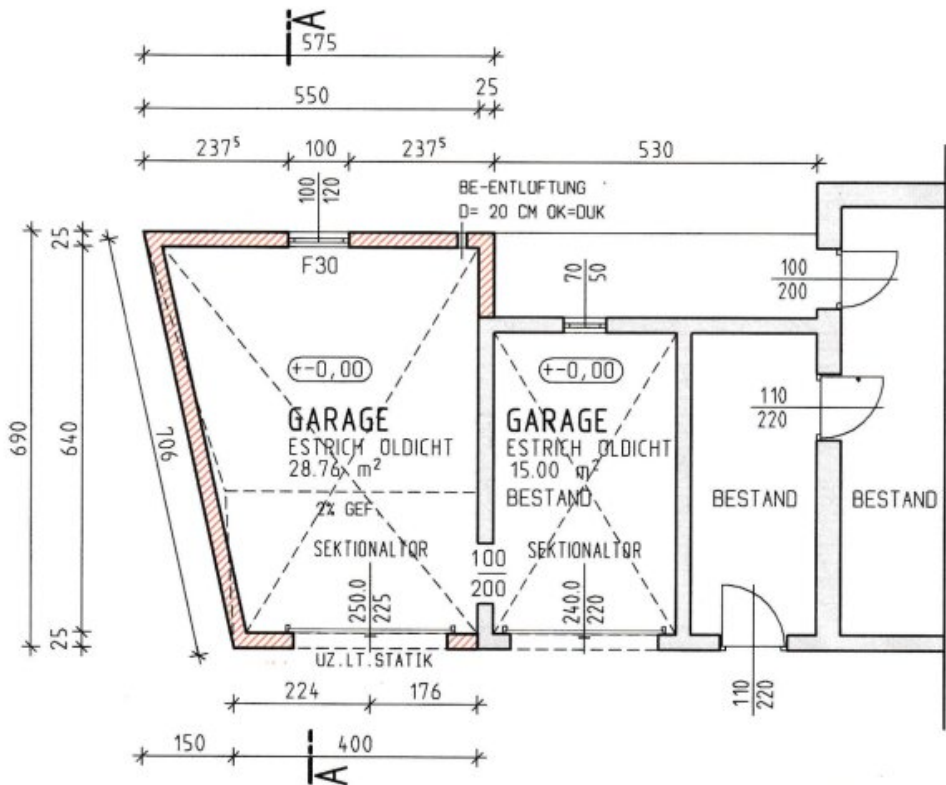
ERDGESCHOSS
