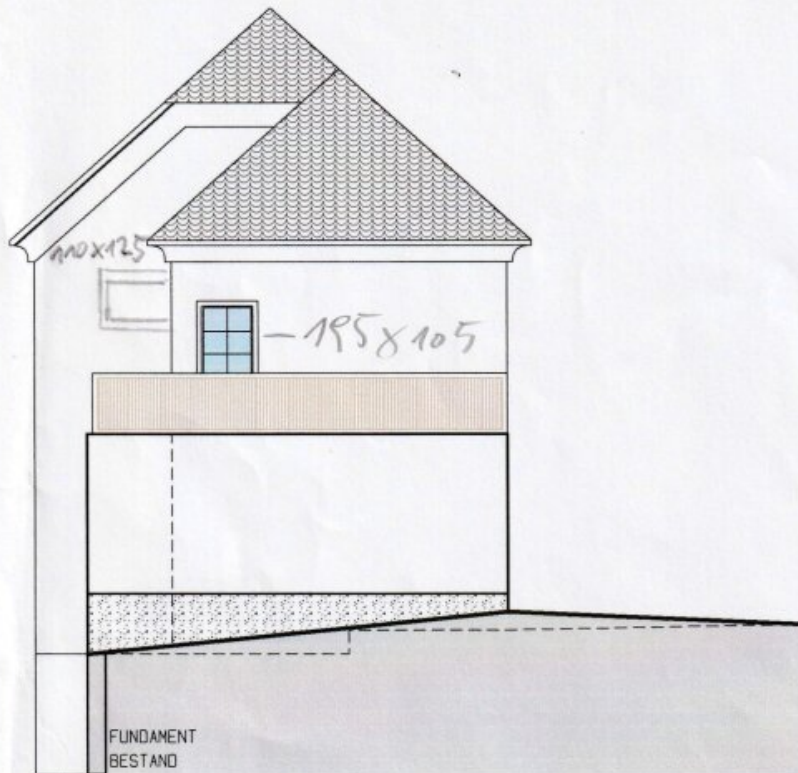
ANSICHT WEST
