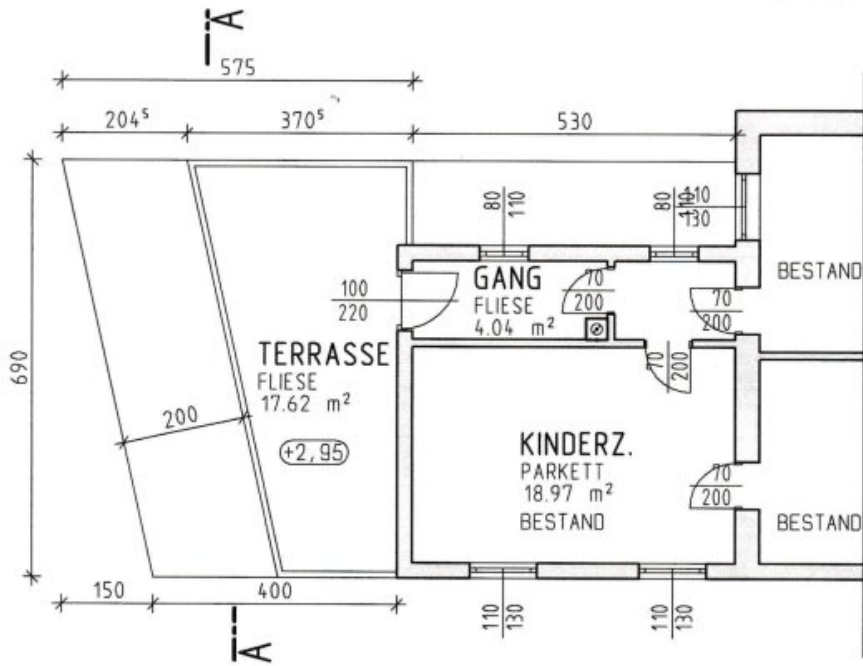
OBERGESCHOSS
