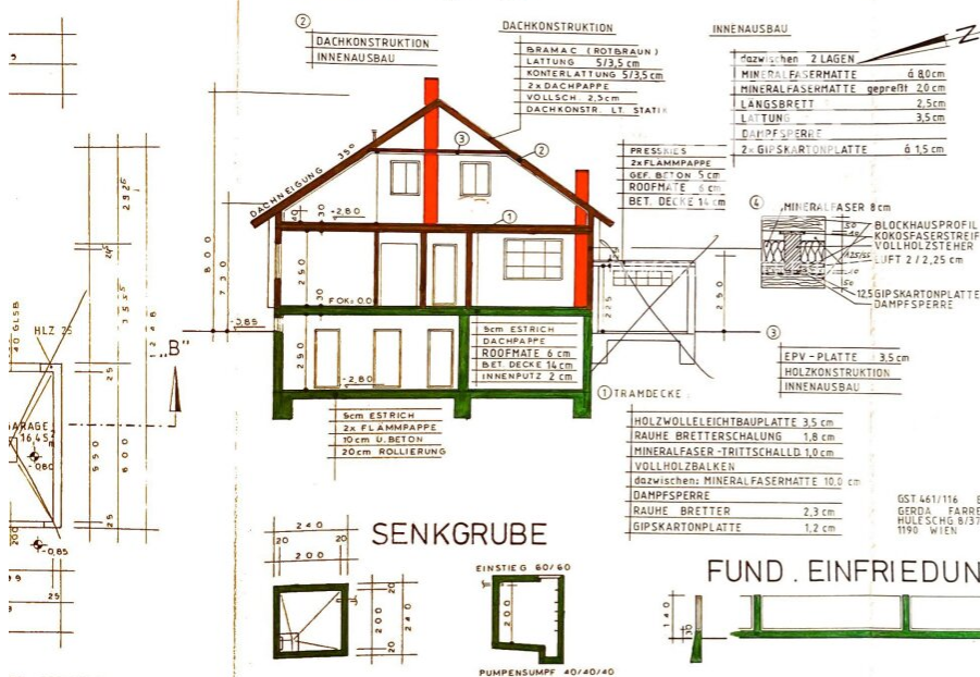
SCHNITT „A“-„B“
