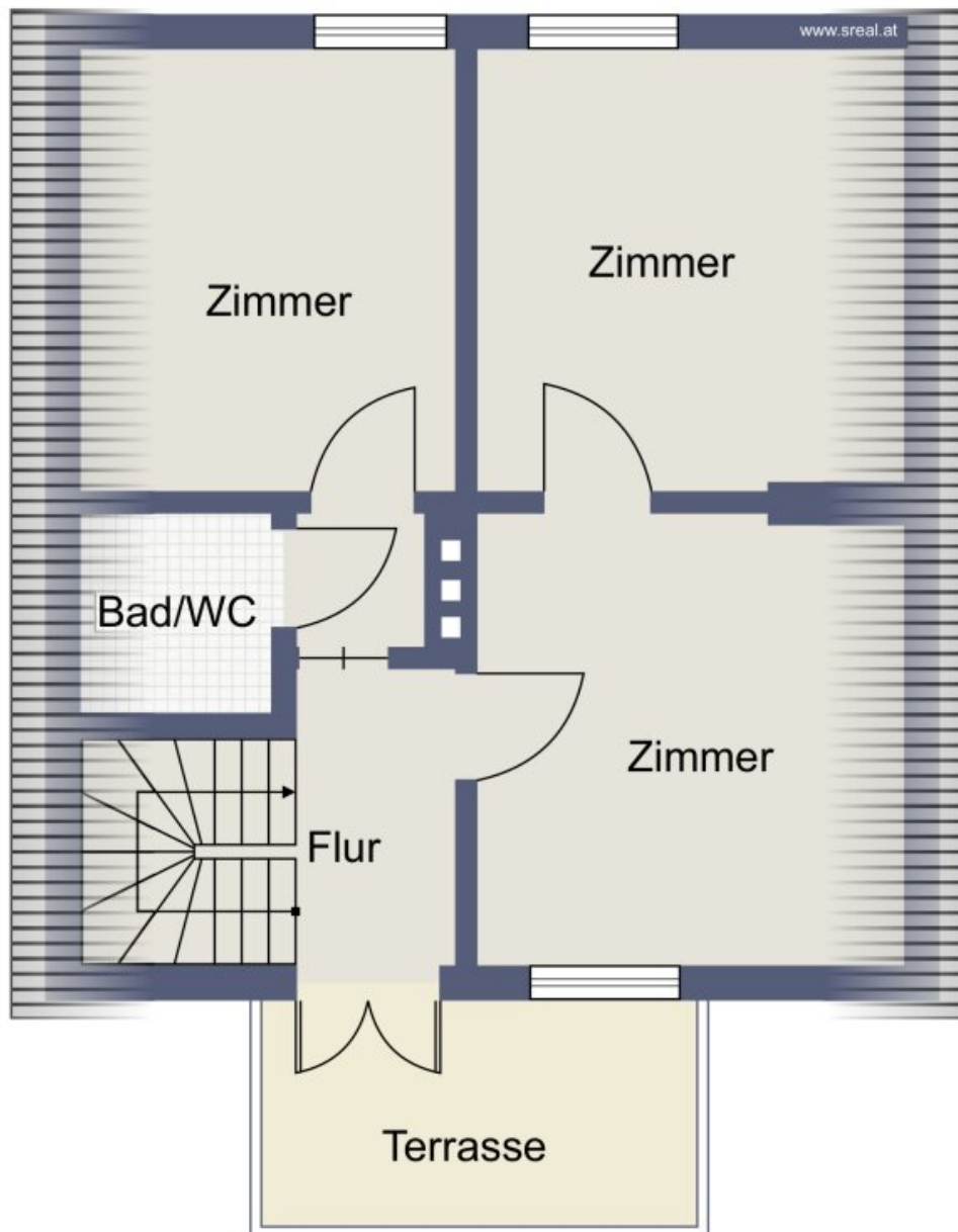
Skizze Dachgeschoss
