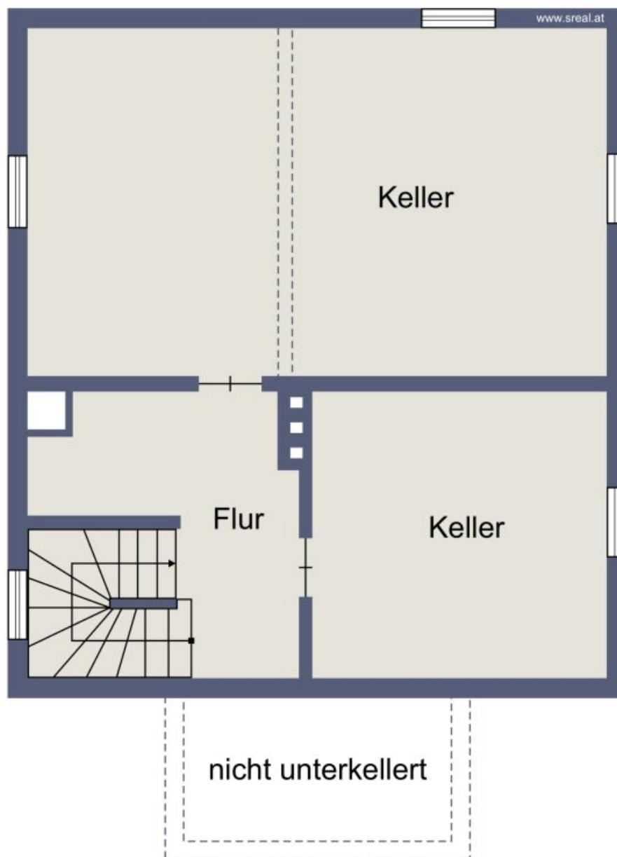
Skizze Kellergeschoss
