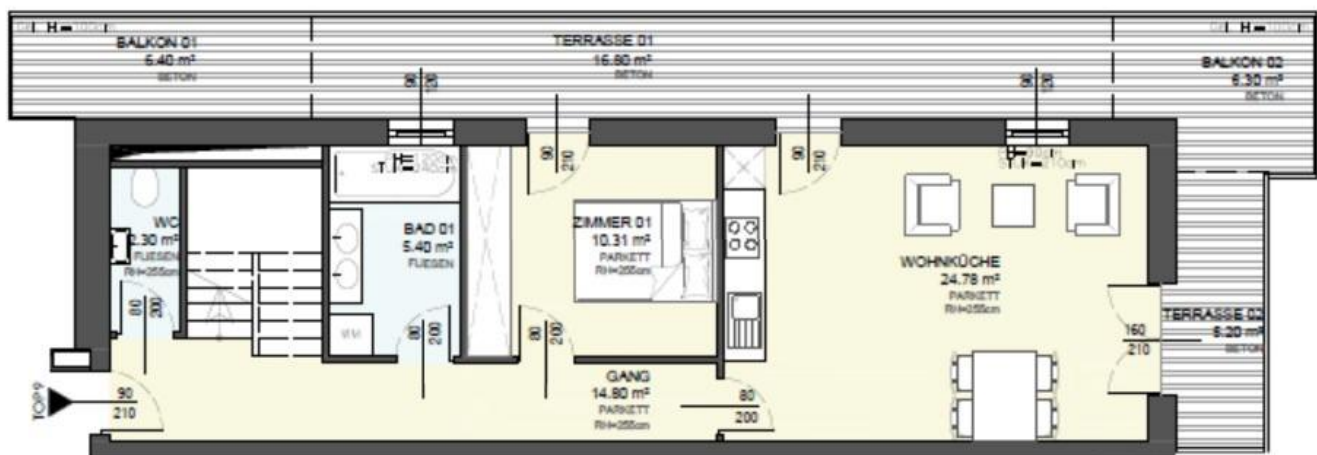
1.DACHGESCHOSS
