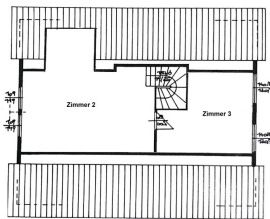
Grundriss-Skizze Obergeschoss
