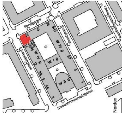
Lageplan 1:500
