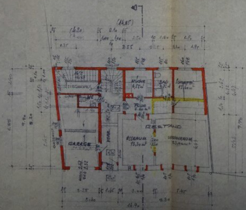
ERDGESCHOSS FELDBAUTE FLÄCHE : 116,63 m² GEBÄUDEFLÄCHE : 87,50 m²
