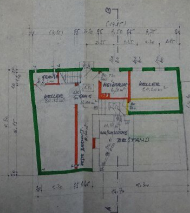
KELLERGECHOSS FELDBAUTE FLÄCHE : 87,50 m²
