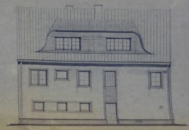
ANSICHT - HOFANSICHT
