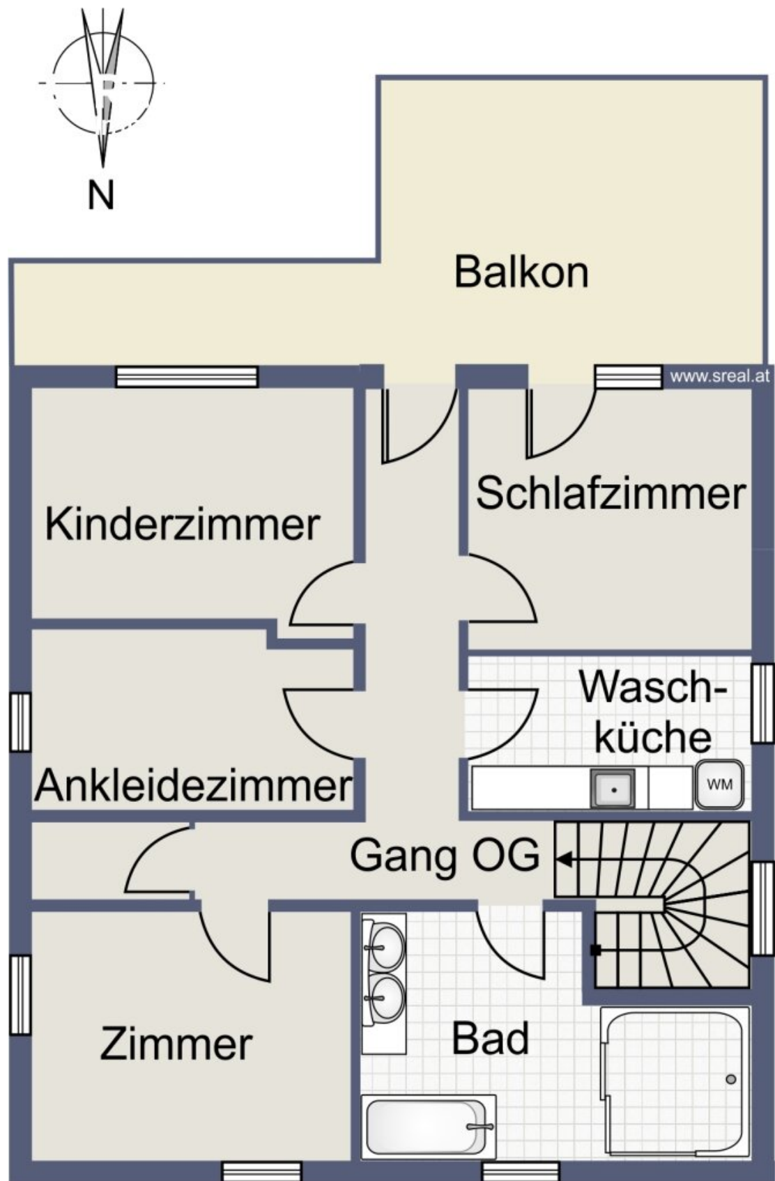
Skizze Obergeschoss
