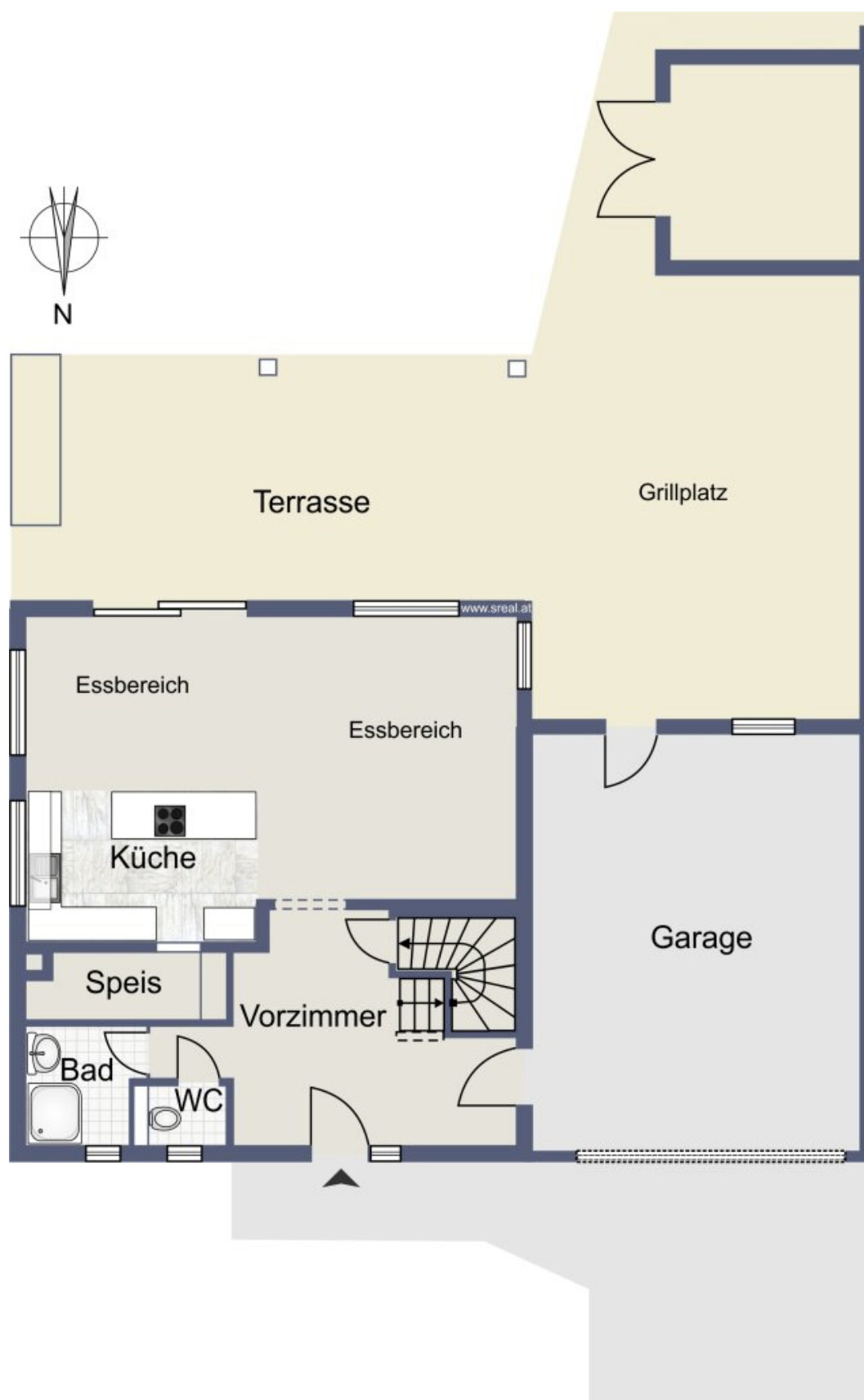
Skizze Erdgeschoss
