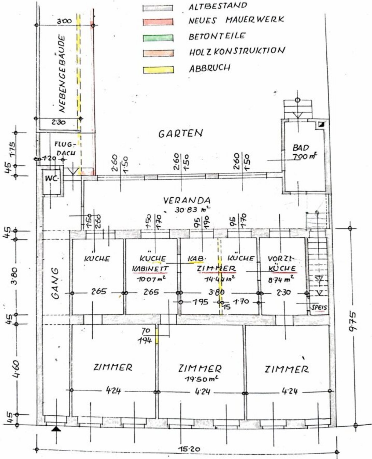
ERDGESCHOSSGRUNDRISS
