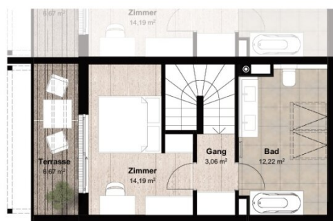
Dachgeschoss M 1:100
