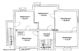
Kellergeschoss Skizze
