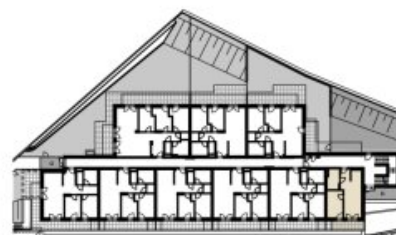
GRUNDRISS BK 03
