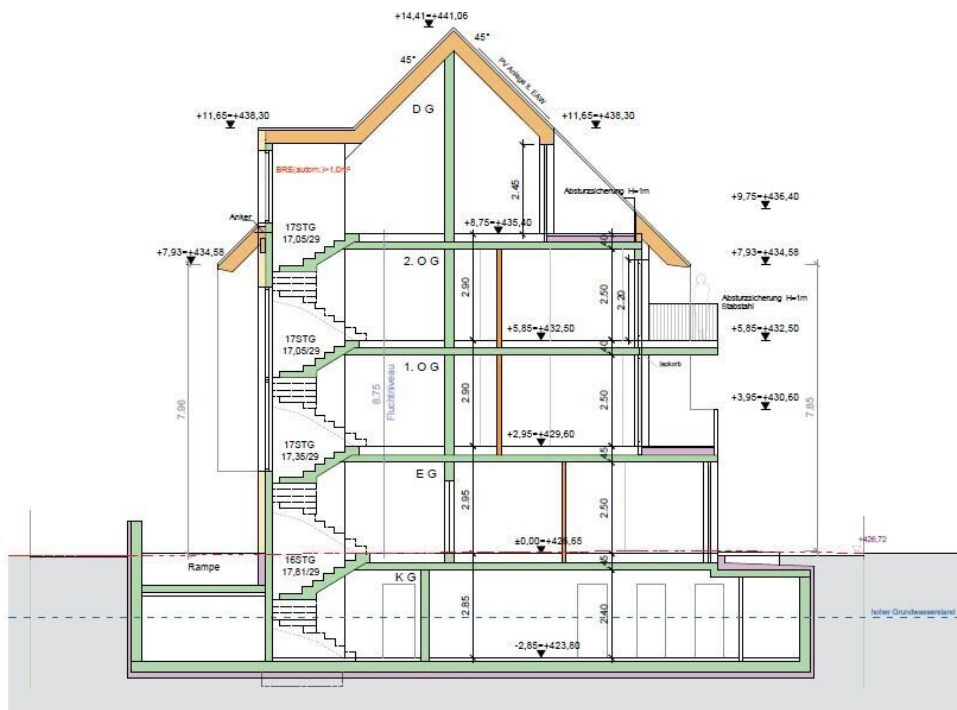
SCHNITT A-A
