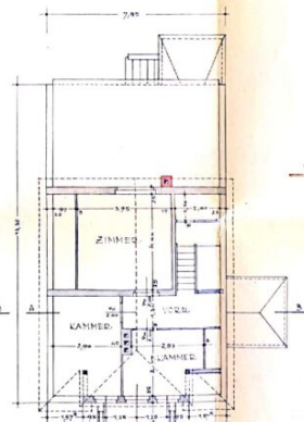
DACHSTOCK
