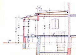
SCHNITT C-D
