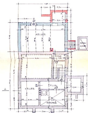
KELLER
