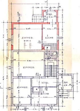
ERDGESCHOSS
