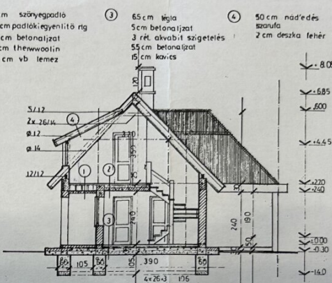
metszet helyszínrajz
