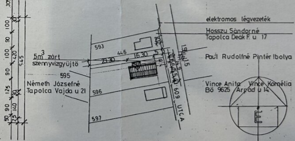
metszet helyszínrajz
