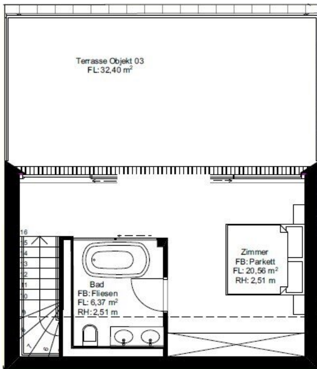
Dachgeschoss 1:100
