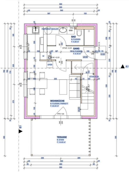
1. ERGESCHOSS 1:50
