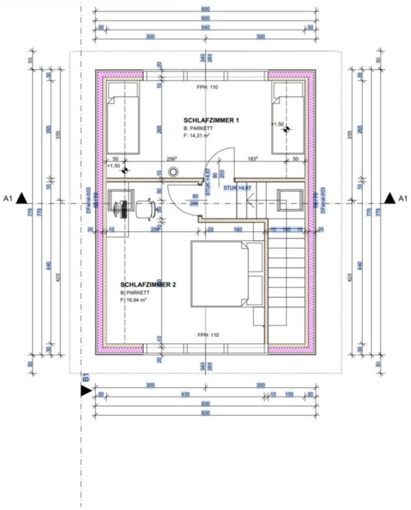
2. OBERGESCHOSS 1:50
