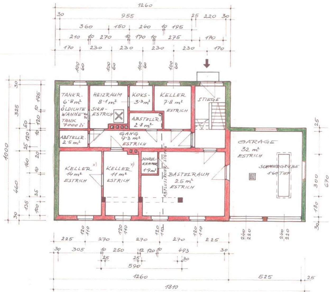
KELLERGESCHOSZ
