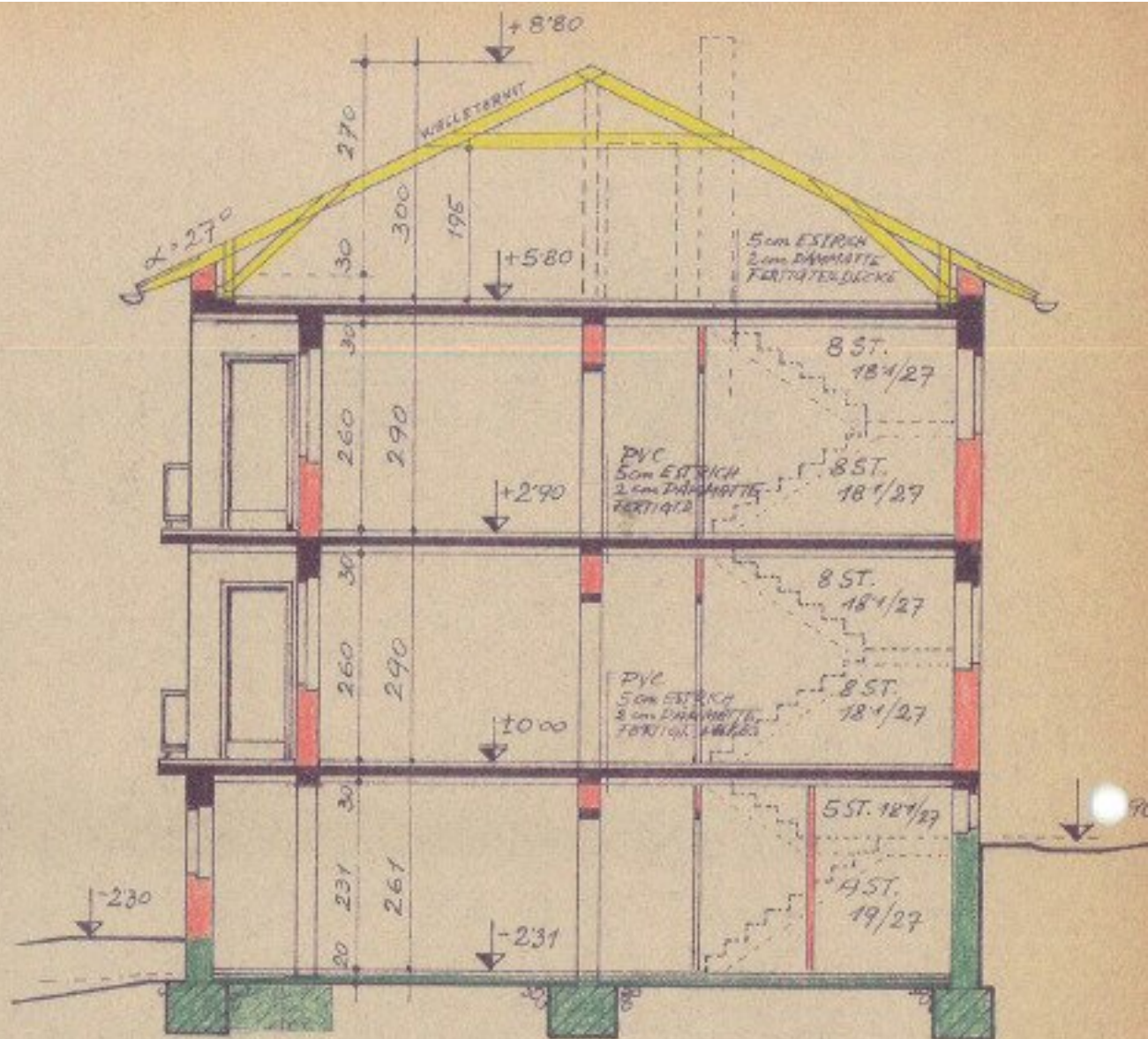
SCHNITT AB
