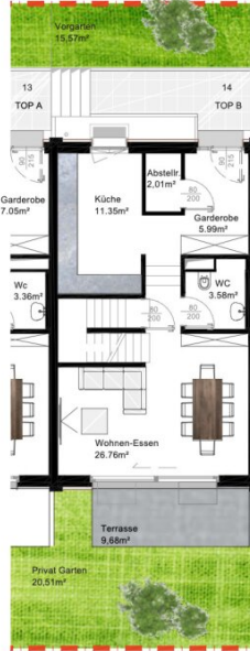
ERDGESCHOSS
