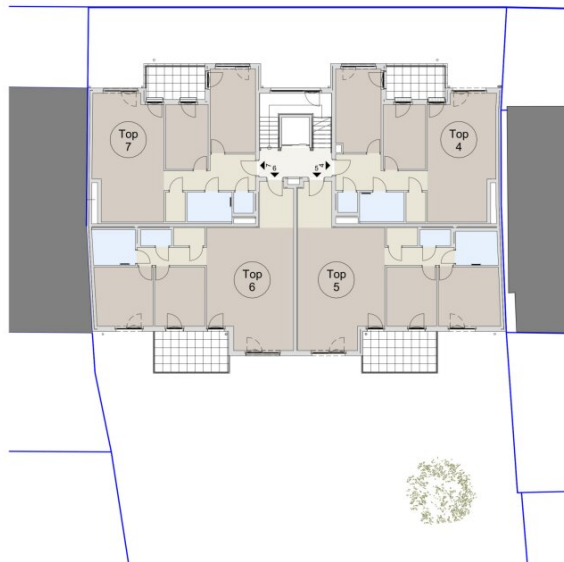
1. STOCK STRASSENBAUKÖRPER 1 : 200
