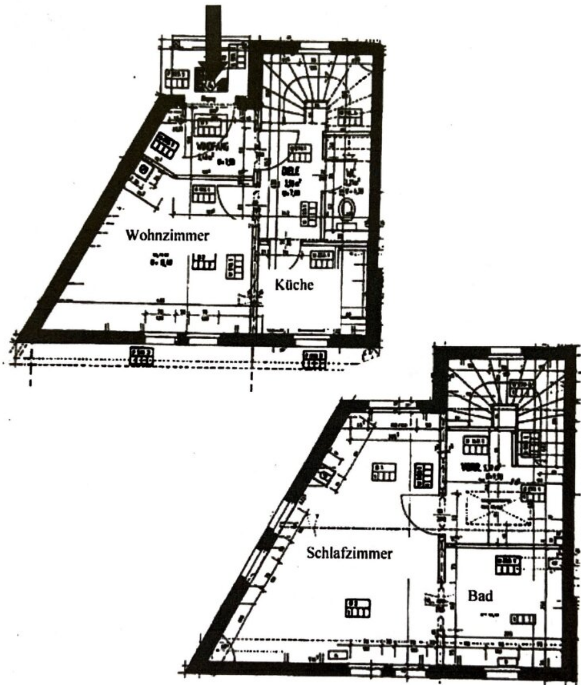
Grundrissplan.jpeg
