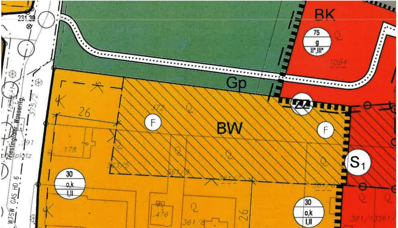
Flächenwidmungs und Bebauungsplan Projektstudie Maria Enzersdorf Schulplatz 1 2344 Maria Enzersdorf
