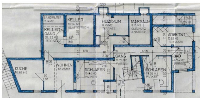
Untergeschoss - Plan weicht teilweise ab, Naturmaße nehmen!
