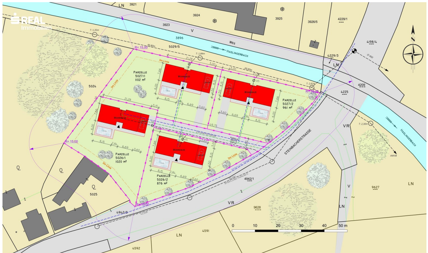
LAGEPLAN
