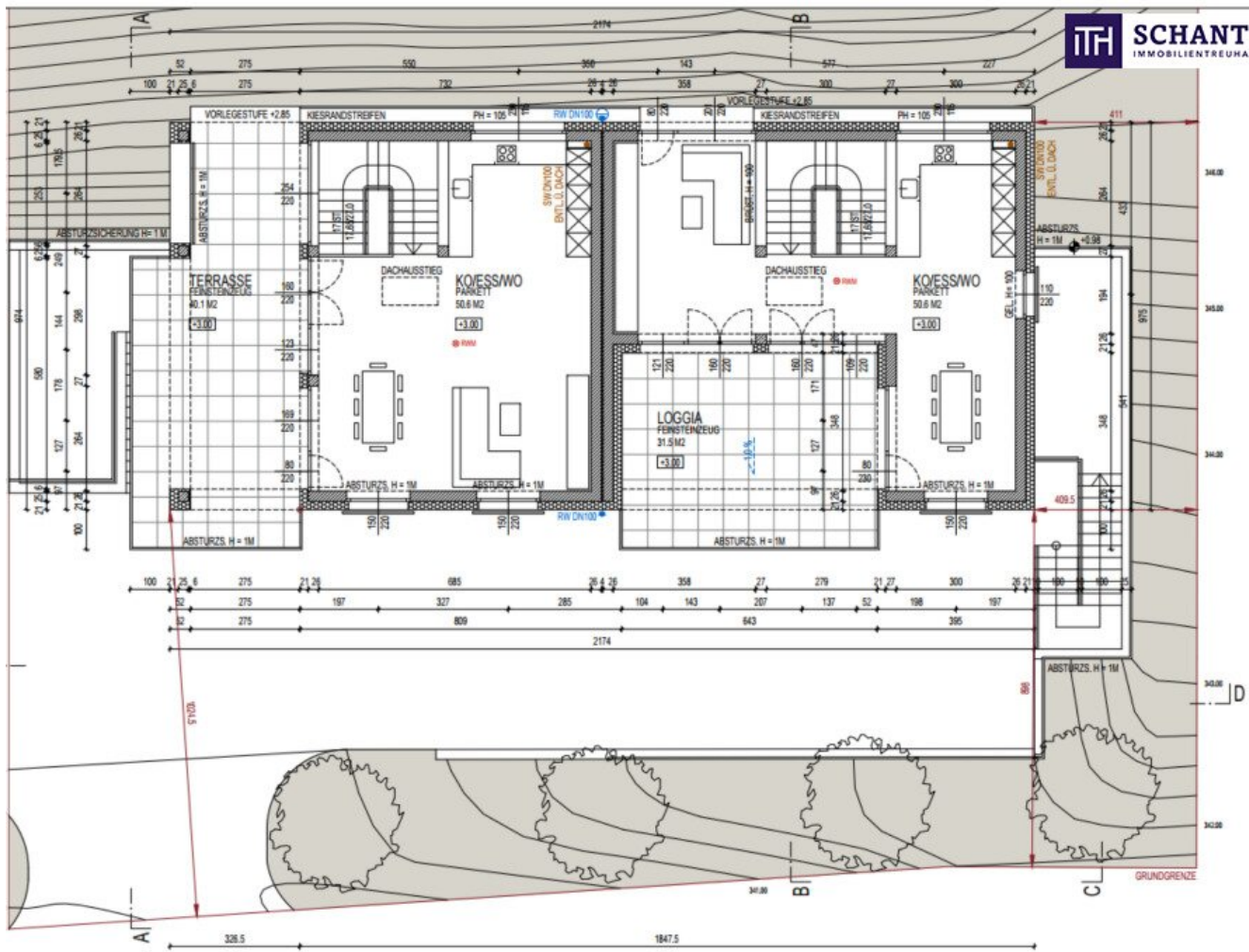
GRUNDRISS OBERGESCHOSS 1:100
