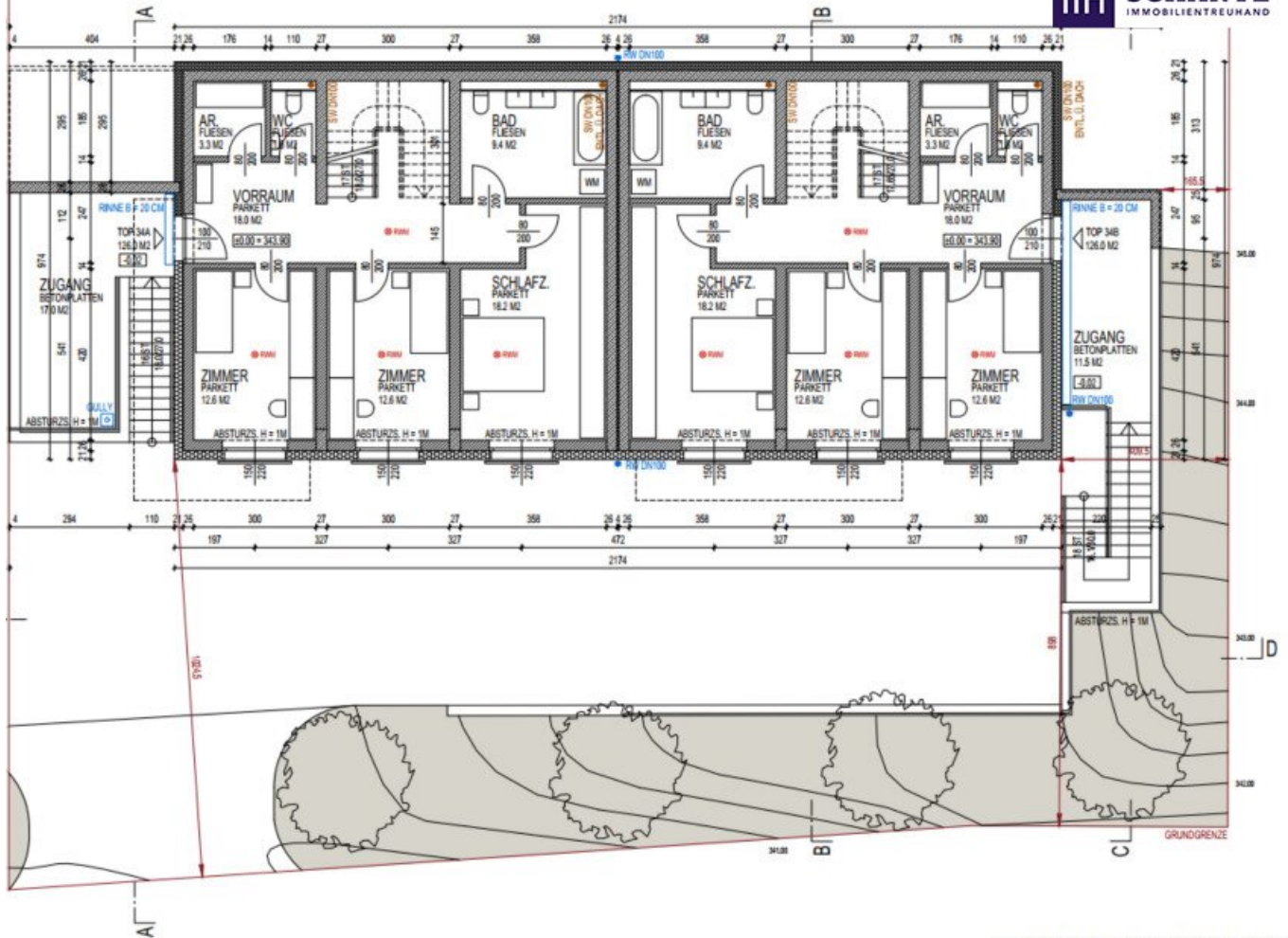
GRUNDRISS ERDGESCHOSS 1:100
