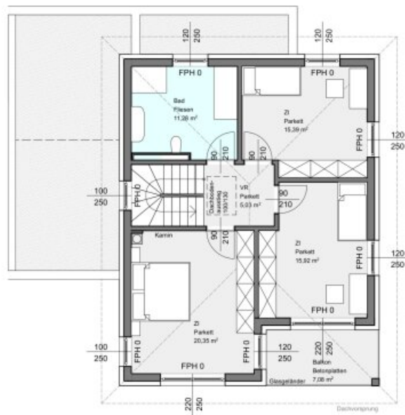
Obergeschoß
