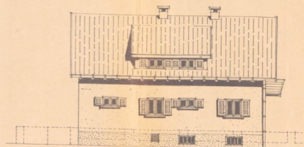
Nordansicht 1:100,
