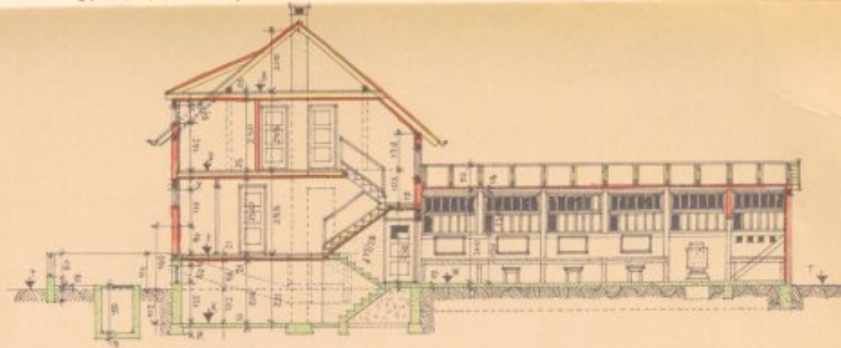
Schnitt A-B 1:100,
