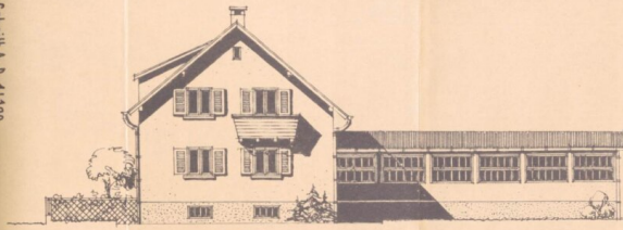
Westansicht 1:100,
