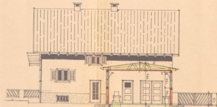
Südsansicht und Schnitt C-D 1:100,
