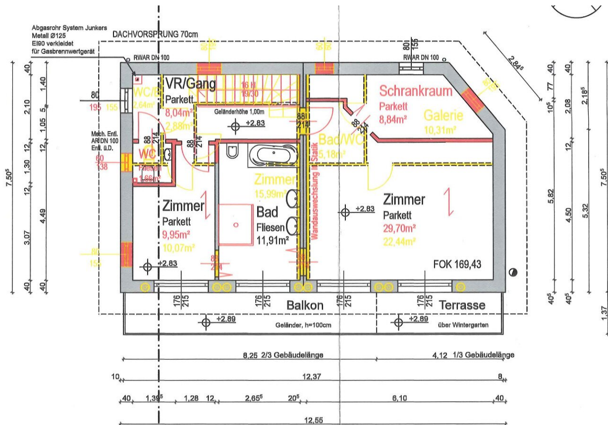
GRUNDRISS OBERGESCHOSS
