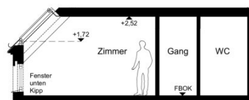
Schnitt
