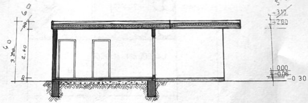
SCHNITT A-B
