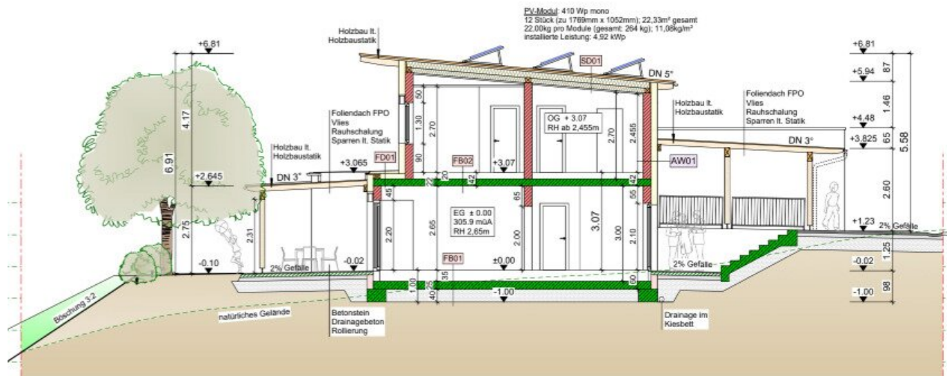
SCHNITT A-A
