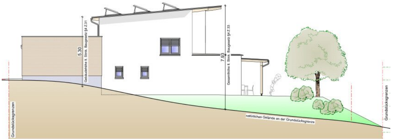
WEST-NORDWESTANSICHT
