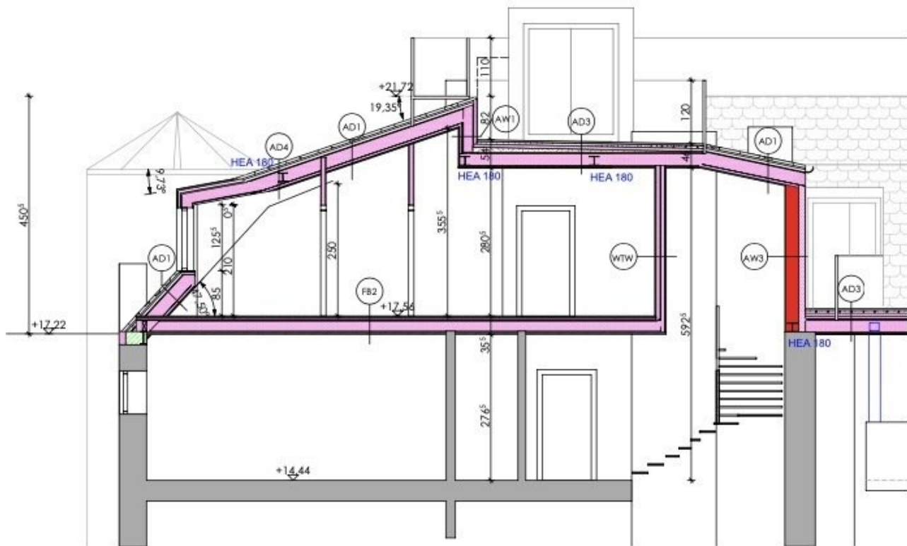
SCHNITT C-C
