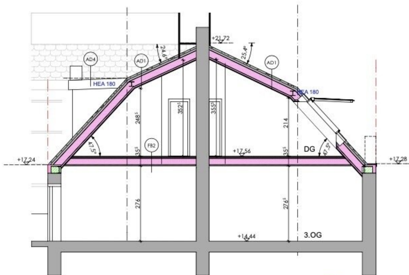
SCHNITT A-A
